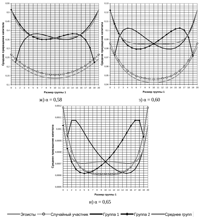
Рис. 1. Ожидаемые приращения капиталов членов групп, эгоистов, случайно выбранных участников за один шаг. Общество: 220 участников, из них 200 эгоистов и 20 членов двух групп; \mu = -1 , \sigma = 60 , порог голосования \alpha варьируется
