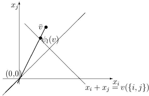
Рисунок 4. Решение \psi_l
