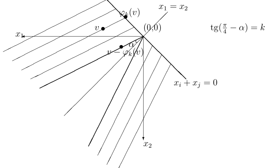
Рисунок 1. Случай k > 0 .
