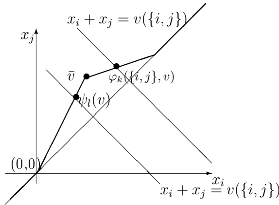
Рисунок 5. Решение \phi_{kl} .
