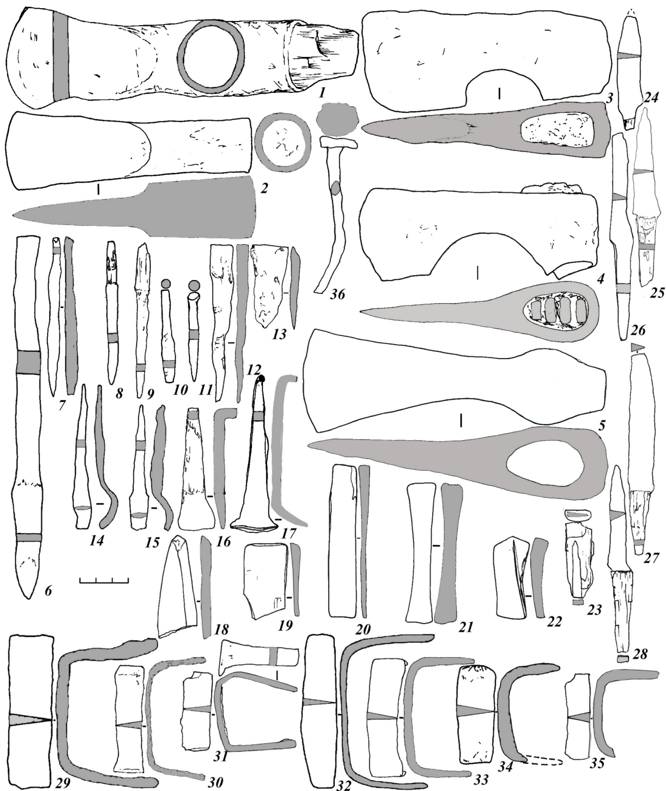
Рис. 2. Орудия деревообработки: 1–5 – топоры, 6–11 – шиповые долота, 12–13 – клинья, 14–15 – резцы-ложжари, 16–17 – пазники, 18–22 – оселки, 23–28 – ножи, 29–35 – наструги, 36 – гвоздь. 1 – п. 59; 2, 10, 17 – п. 234а; 3, 34 – п. 78; 4, 9, 12, 15, 20, 36 – п. 216; 5 – п. 2796, 6, 32 – п. 65; 7, 23, 31 – п. 242; 8, 14, 24 – п. 120; 11, 19, 27 – п. 247; 13 – п. 169; 16, 26, 33 – п. 234а, жертвенный комплекс; 18, 28, 35 – п. 250; 21–22 – п. 242, жертвенный комплекс; 25, 30 – п. 249; 29 – п. 61
