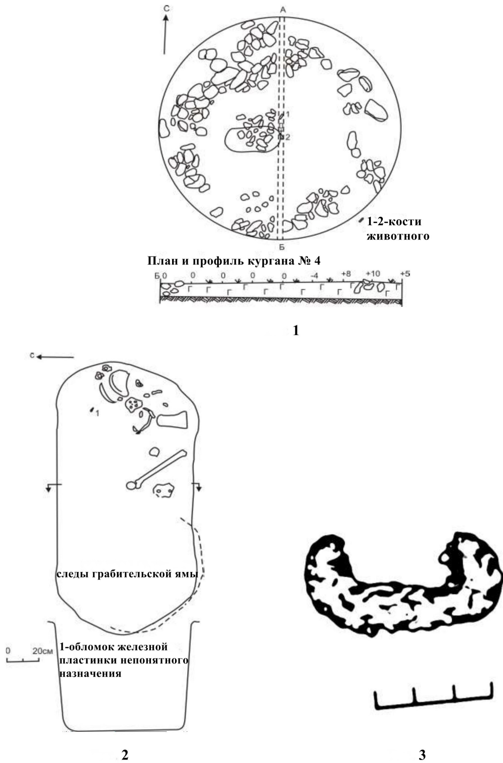
Рис. 4. 1 – план и профиль кургана № 4; 2 – план разграбленного погребения в кургане № 4; 3 – обломок калачевидного кресала
