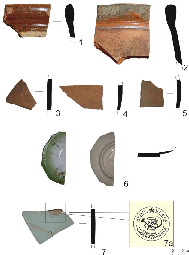
Рис. 3. Республика Башкортостан, город Уфа, ул. Театральная, 3. Археологический материал выявленный в ходе проведения археологического наблюдения (керамика):
