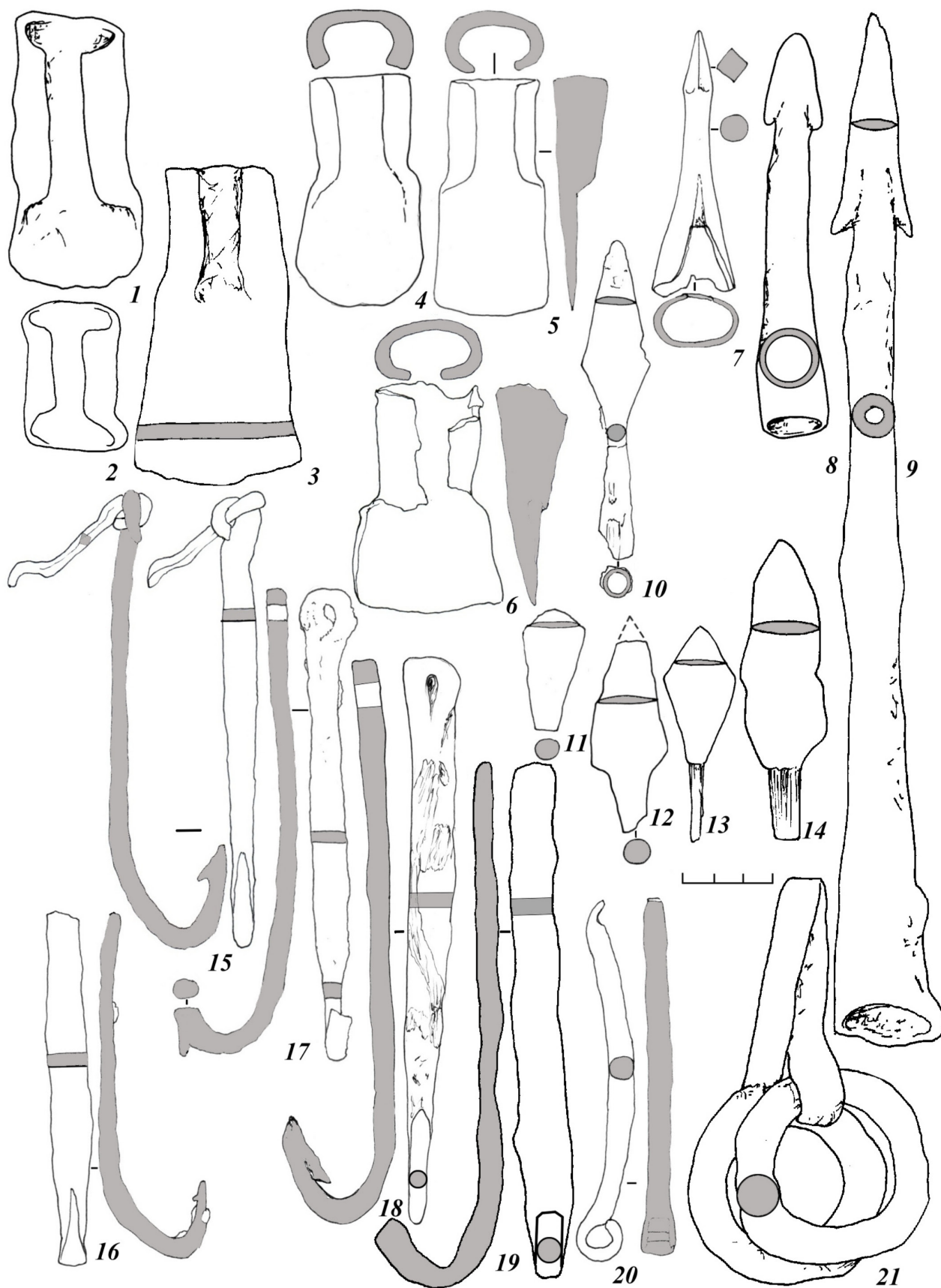
Рис. 3. Хозяйственные орудия: 1–6 – наконечники мотыг, 7–9 – наконечники копий, 10–14 – наконечники стрел, 15–19 – рыболовные крюки, 20–21 – фрагменты удил. 1, 8 – п. 78; 2, 13 – п. 120; 3, 9 – п. 61; 4, 12 – п. 1796; 5 – п. 242; 6, 15 – п. 249; 7 – п. 242, жертвенный комплекс; 10–11 – п. 234а; 14, 19, 21 – п. 65; 16, 20 – п. 250; 17 – п. 247; 18 – п. 169
