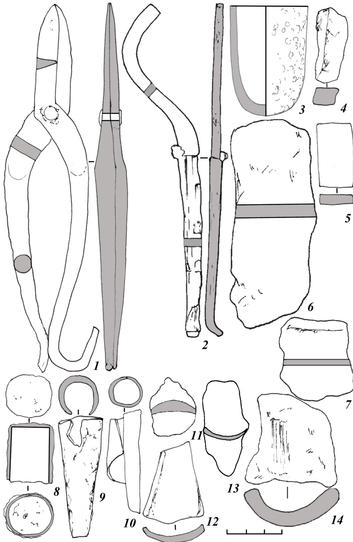
Рис. 4. Ремесленные инструменты и фрагменты изделий: 1 – ножницы по металлу, 2 – шабер, 3 – тигель, 4–7 – железные бруски (кузнечные заготовки?), 8–14 – фрагменты втулок. 1–2, 10, 12 – п. 234а, жертвенный комплекс; 3, 8 – п. 242; 4, 9 – п. 169; 5 – п. 242, жертвенный комплекс; 6 – п. 59; 7 – п. 78; 11, 14 – п. 61; 13 – п. 120
