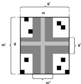
Рис. 1. оп-бикластер
