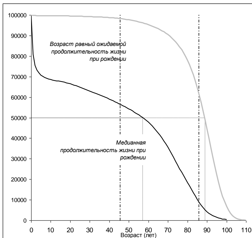
Рис. 1. Функция дожития
