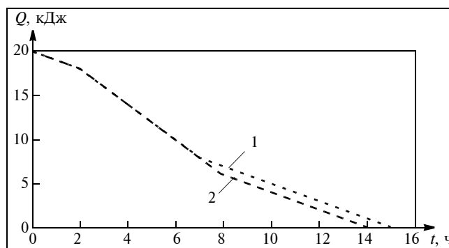
Рис. 3. Зависимости остаточной энергии на узлах от времени работы в сетях при различных методах передачи аудиоданных:
