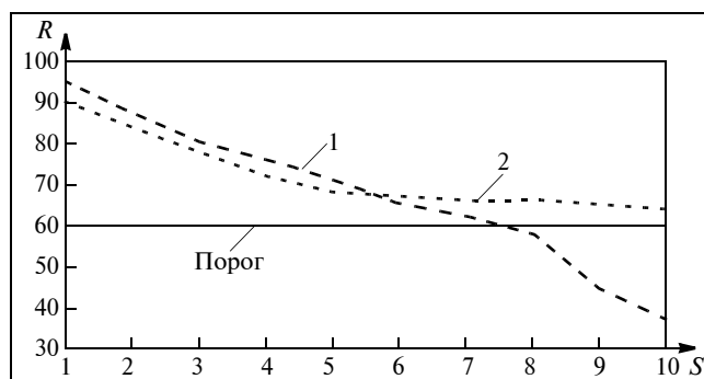
Рис. 2. Зависимость качества предоставляемого сервиса от числа потоков в сетях:
