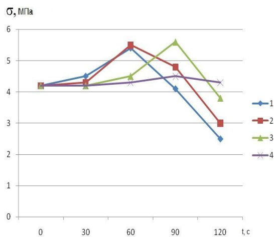
Рисунок 2. Изменение условной прочности ( \sigma ) при растяжении армированных (а) и неармированных (б) повторных вулканизатов от времени ( t ) воздействия СВЧ энергии при различных режимах обработки: 1 — ДВ 100, 2 — ДВ 75, 3 — ДВ 60, 4 — ДВ 45.
