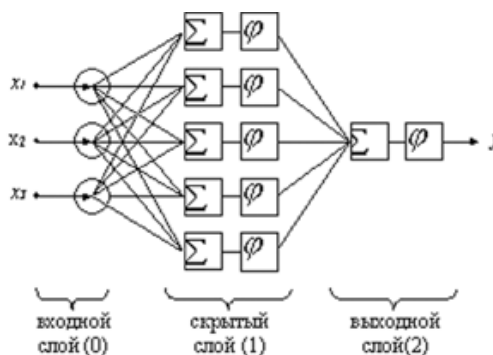
Рис. 2. Искусственная нейронная сеть
