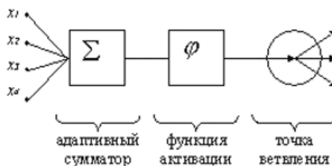
Рис. 1. Формальный нейрон
