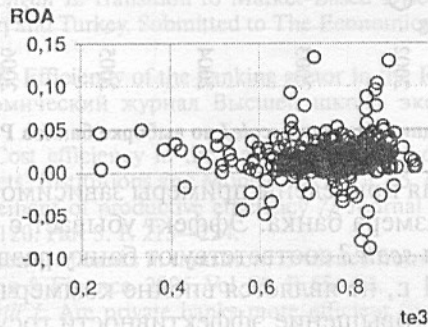
Рис. 1. Диаграмма te3-ROA
