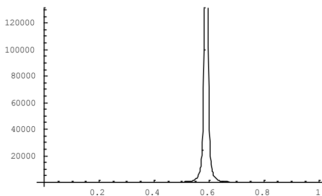
Рис. 3. Перколяция глобальной системы «деньги-долг».
