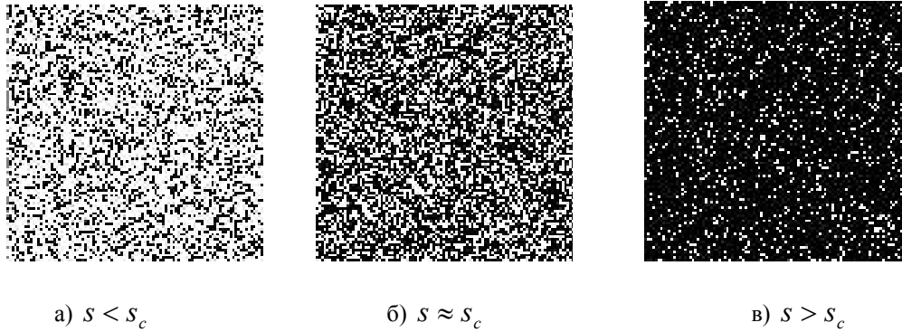
Рис.27.1. Конфигурации сети участников рынка размера L = 100 для разных объемов ликвидности.
