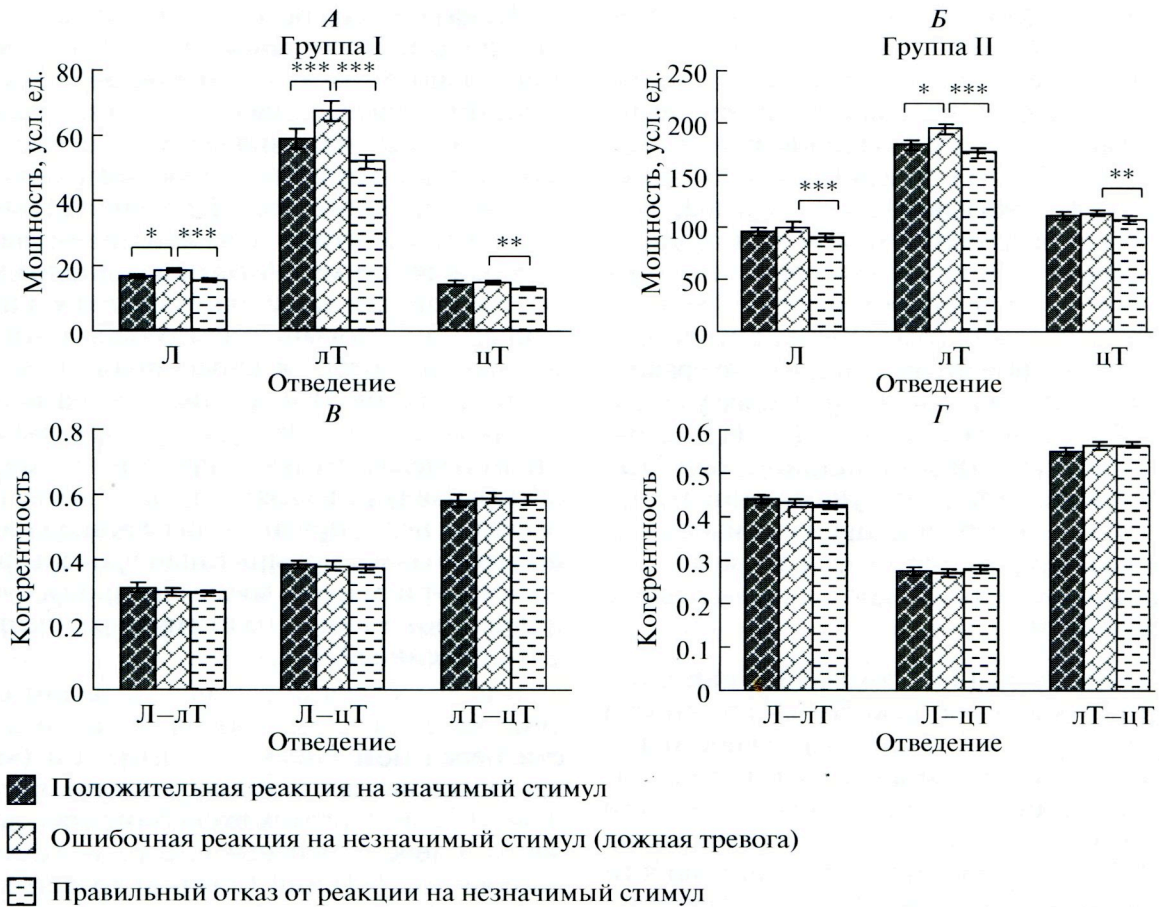
Рис. 3. Фоновая гамма-активность перед предъявлением стимулов при положительной инструментальной реакции, ошибочной реакции и правильном отказе от реакции. А, Б – мощность гамма-активности в группах I ( n = 13 ) и II ( n = 27 ), В, Г – когерентность гамма-активности в группах I ( n = 13 ) и II ( n = 27 ). Остальные обозначения как на рис. 1.
