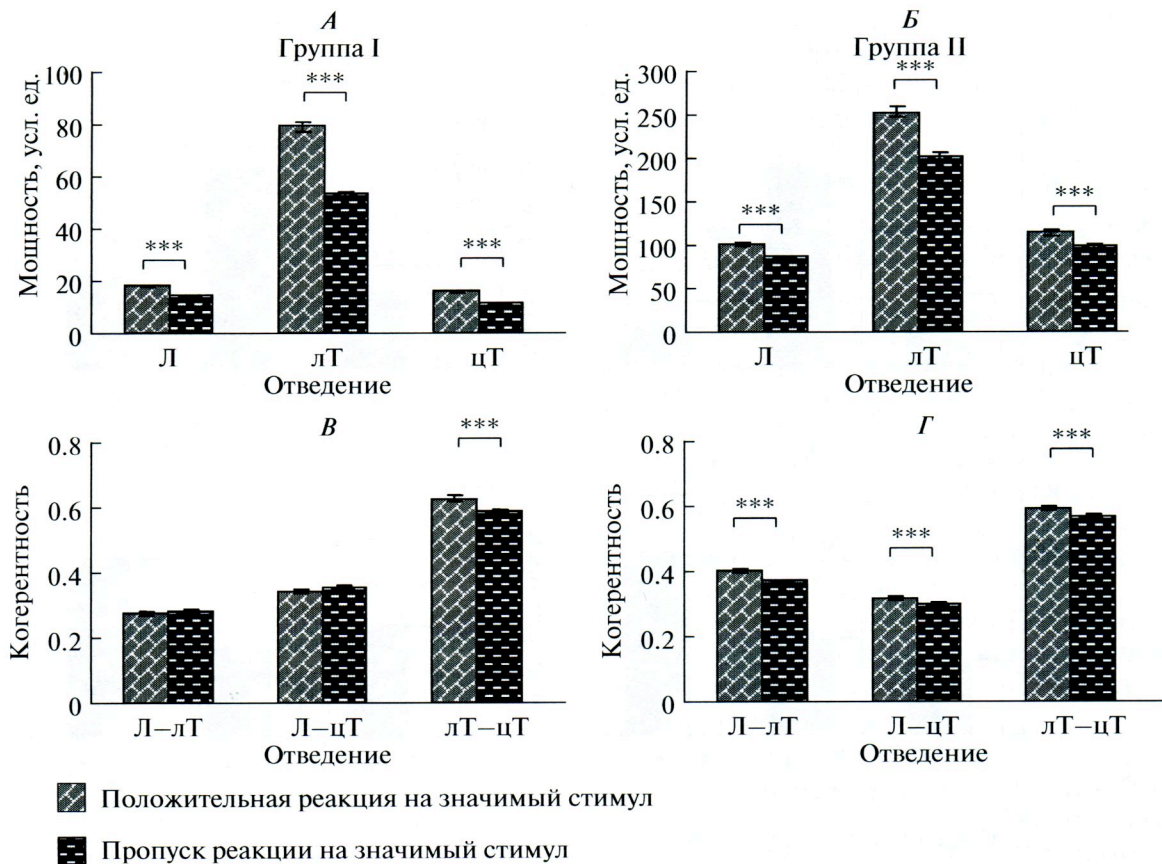
Рис. 2. Фоновая гамма-активность перед предъявлением значимых стимулов при положительной инструментальной реакции и при ее пропуске. A, Б – мощность гамма-активности в группах I ( n = 50 ) и II ( n = 84 ), B и Г – когерентность гамма-активности в группах I ( n = 50 ) и II ( n = 84 ). Остальные обозначения как на рис. 1.
