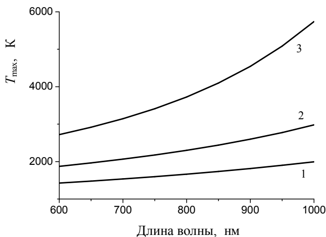
Рис. 2. Спектральная зависимость максимальной температуры, которую можно определить с помощью спектрометра с динамическим диапазоном 1300, не меняя условий эксперимента (т. е. при фиксированном времени накопления спектра и неизменной оптической схеме измерений). Минимальная температура (К): 1000 (1), 1200 (2), 1500 (3)
