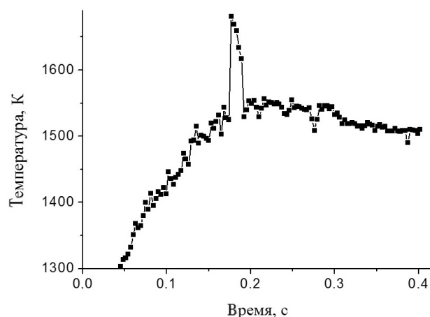
Рис. 3. Зависимость температуры стальной пластинки толщиной 0.26 мм от времени после начала облучения лазерным пучком (мощность 12 Вт)
