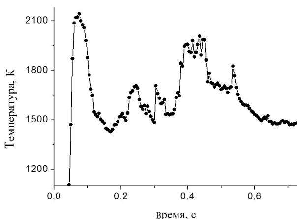
Рис. 4. Зависимость температуры слоя титановых шариков диаметром 50 мкм от времени после начала облучения лазерным пучком (мощность 6 Вт)
