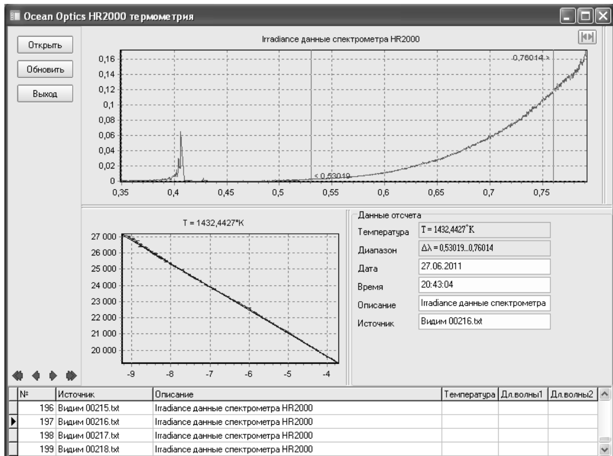
Рис. 1. Окно программы для обработки последовательности спектров теплового излучения и вычисления температур.
