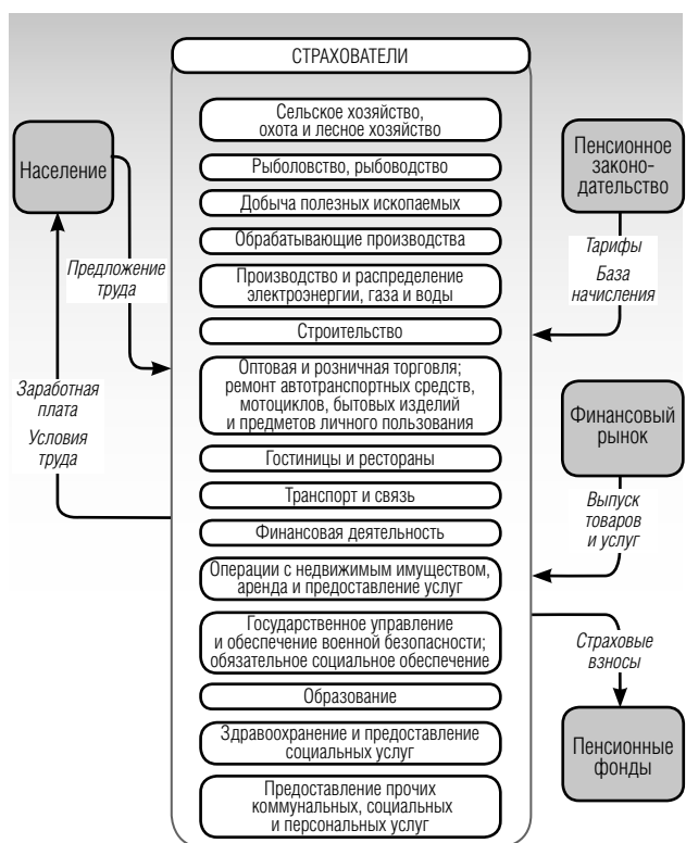
Рис. 5. Подсистема «Страхователи»
