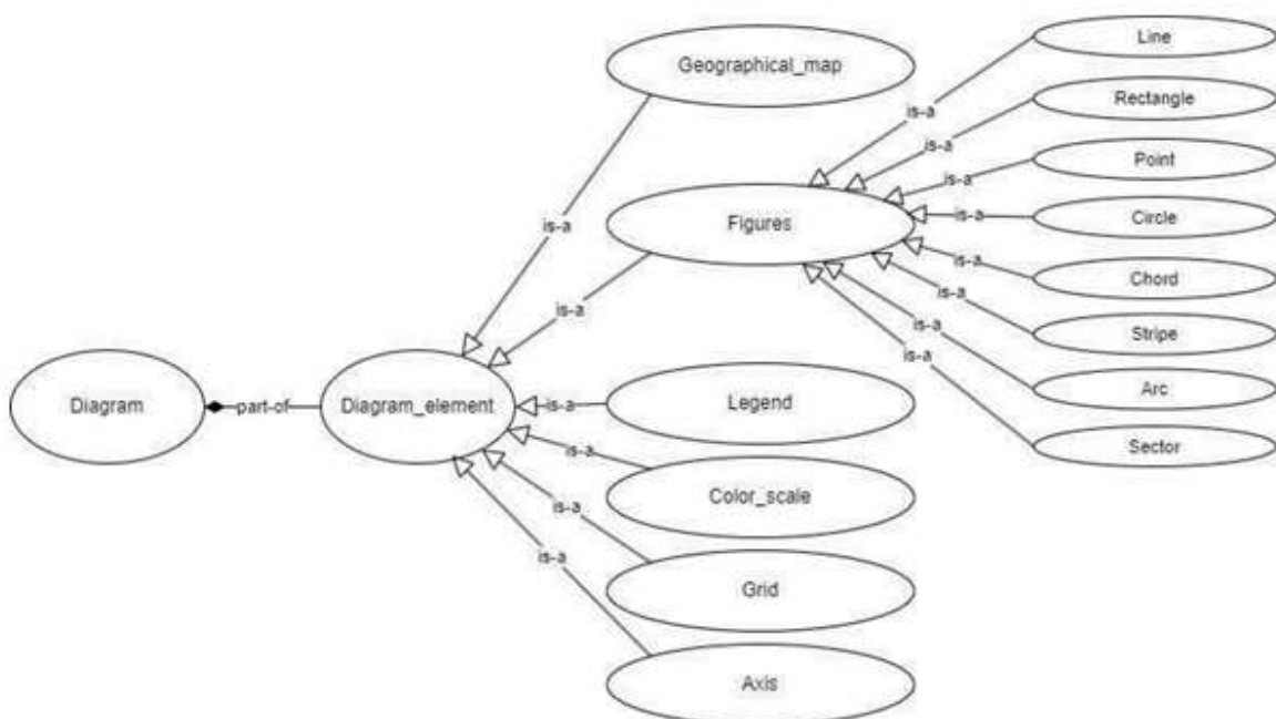
Рис. 6. Фрагмент многоаспектной онтологии: иерархия классов элементов диаграммы в онтологии
