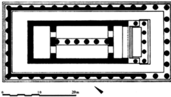
Рис. 5. Д. Мертенс. План храма В в Метапонте ок. 530 г. до н.э. Воспроизводится по: [21, p. 791 No. 33.8.2.3b]
