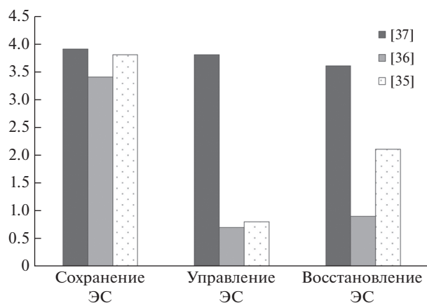
Рис. 2. Поглощение парниковых газов в разных типах лесоклиматических проектов с себестоимостью ниже 45 долл. за углеродную единицу для удержания глобального потепления ниже 2°C, Гт CO 2 -экв./год. По данным [35–37]
