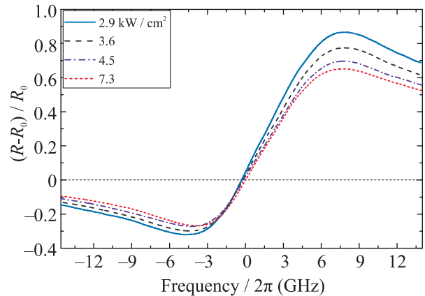
Рис. 1. (Цветной онлайн) Относительный коэффициент селективного отражения для значений интенсивности I = 2.9, 3.6, 4.5, 7.3 кВт/см ^2 в зависимости от частоты падающего излучения
