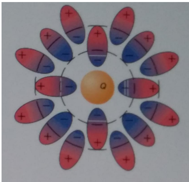
Рис. 29. Экранировка заряда поляризационными вакуумными диполями
