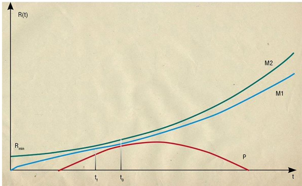
Рис. 10. Три возможных главных сценария эволюции космоса, предложенных Фридманом в 1922 г., изображены в виде зависимости космического радиуса от времени. В первом монотонном сценарии, M1, Вселенная расширяется из сингулярности с уменьшающейся скоростью до некоторого момента t_f , затем скорость расширения увеличивается. Настоящее время отмечено на графике линией, проходящей через t_0 . Сценарий M1 наилучшим образом согласуется с современными астрофизическими наблюдениями. Кривая M2 соответствует сценарию, когда Вселенная начинает расширяться из состояния с ненулевым начальным радиусом R_{min} . Периодический сценарий P соответствует расширению из точки и сжатию обратно в точку. (Physics Today. October 2012. P. 38)
