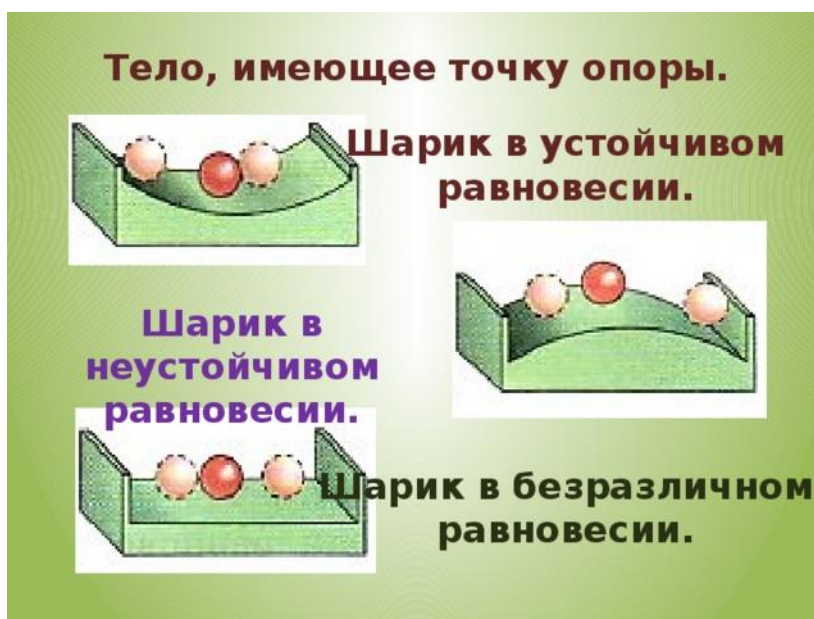
Рис. 38. Различные состояния равновесия шарика
