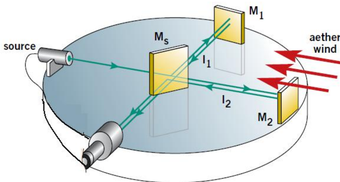
Рис. 24. Упрощенная схема эксперимента Майкельсона-Морли
