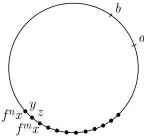
Рис. 1.9. Пример 3
