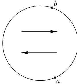
Рис. 1.10. Пример 4
