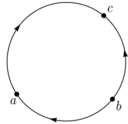
Рис. 1.8. Пример 1
