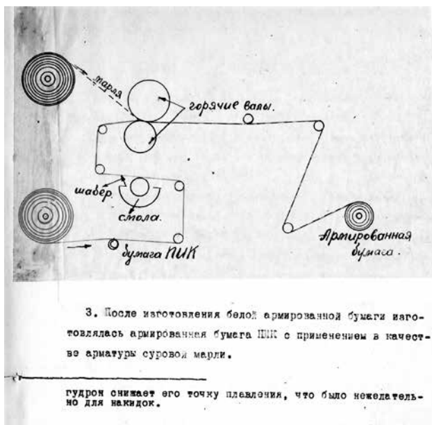
Фото 1. Схема машины для нанесения покрытия при производстве армированной бумаги
