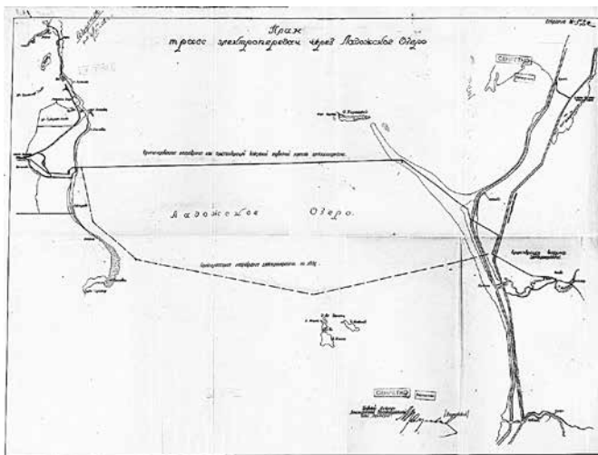
Фото 10. План трасс электропередач через Ладожское озеро, 4 ноября 1942 г.
