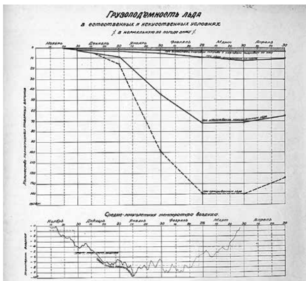
Фото 2. График грузоподъемности льда в естественных и искусственных условиях
