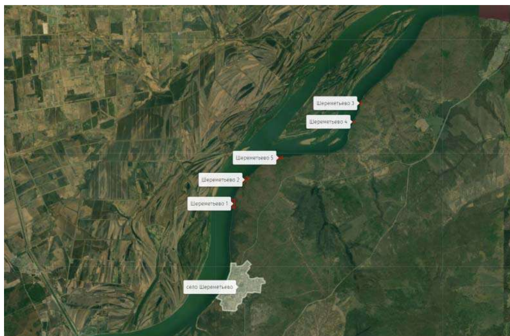
Рис. 1. Карта местонахождений петроглифов Шереметьево в Хабаровском крае Fig. 1. Map of the locations of the Sheremet'yevy petroglyphs in the Khabarovsk Territory
