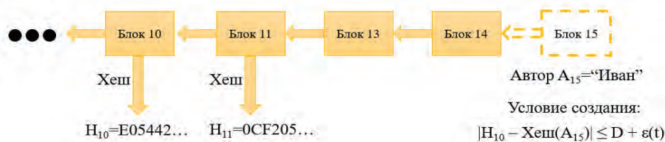
Рис. 3. Пример согласования транзакции
