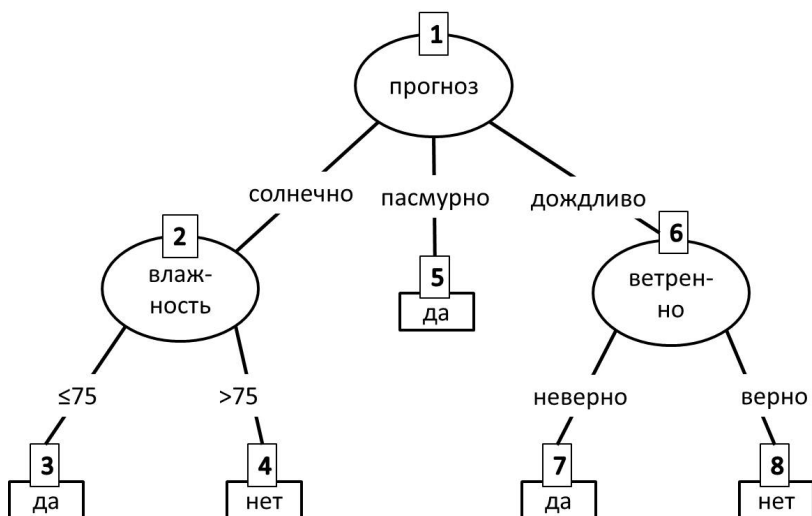
Рис. 1. Базовый пример дерева решений для пакета partykit
