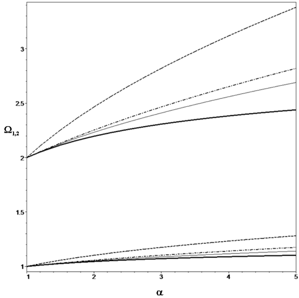
Рис. 1: Частоты \Omega_{1,2} основной и первой мод, как функции параметра \alpha .
