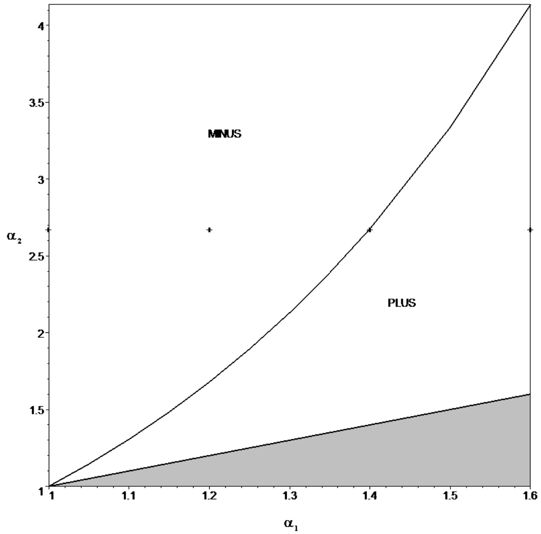
Рис. 5: График кривой F(\alpha_1, \alpha_2) = 0 , где \alpha_1, \alpha_2 – значения, при которых точка минимума амплитуды колебаний первой моды (34) равна -0.5z/L . Поле MINUS – отрицательные смещения, PLUS – положительные. Знаком «+» отмечены параметры, для которых построены графики рис. 6. Затененная область \alpha_1 > \alpha_2 .
