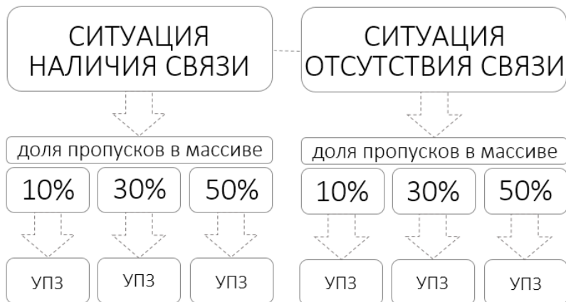
Рис. 4. Результаты сравнения эффективности правила Рубина и усреднения подставленных значений для вычисления коэффициента корреляции Пирсона
