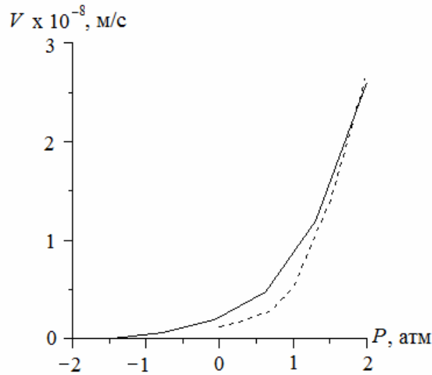
Рис. 3. Графики зависимости скорости потока на срезе корня от разности гидростатических давлений между окружающей средой и ксилемой (пунктирная линия соответствует экспериментальным данным, сплошная – расчетам на основе модели)
