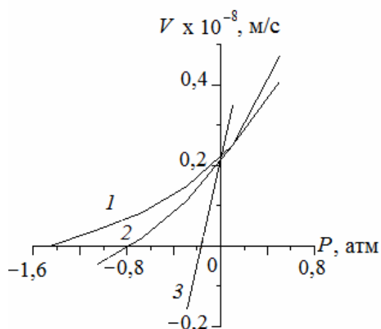
Рис. 4. Графики зависимости скорости потока на срезе корня от разности гидростатических давлений между окружающей средой и ксилемой при различных проницаемостях поясков Каспари по отношению к растворенному веществу и фиксированной гидравлической проводимости \Omega = 2,9 \cdot 10^{-15} м·Па -1 ·с -1 . Кривая 1 получена для непроницаемых поясков Каспари; 2 — при \Lambda = 2 \cdot 10^{-10} м·с -1 , \sigma_c = 0,6 ; 3 — при \Lambda = 3,4 \cdot 10^{-10} м·с -1 , \sigma_c = 0,1
