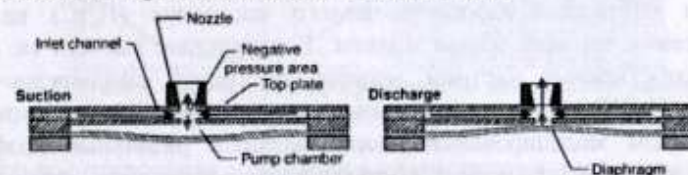
Рисунок 1. Вид мембранного пьезонасоса
