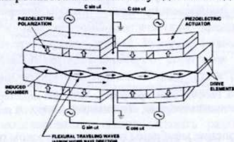
Рисунок 6. Схема возбуждения пьезокерамики с продольным пьезомодулем d_{33}
