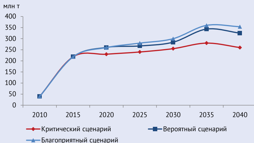
Рисунок 2.53 – Прогноз добычи сланцевой нефти США по трем сценариям
