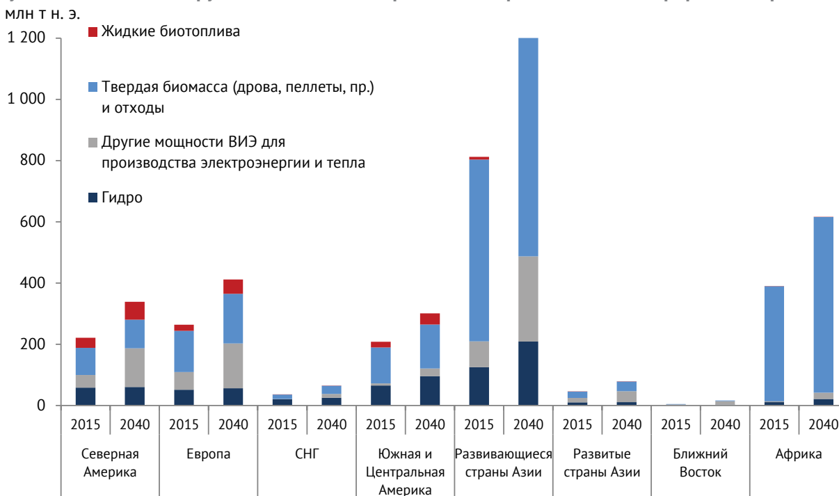
Рисунок 2.32 – Доминирующие виды ВИЭ по регионам мира и показатели прироста потребления
