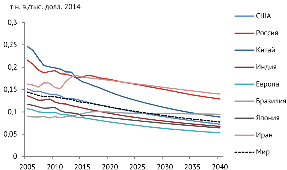
Рисунок 2.2 – Энергоемкость ВВП по миру и отдельным странам в Вероятном сценарии
