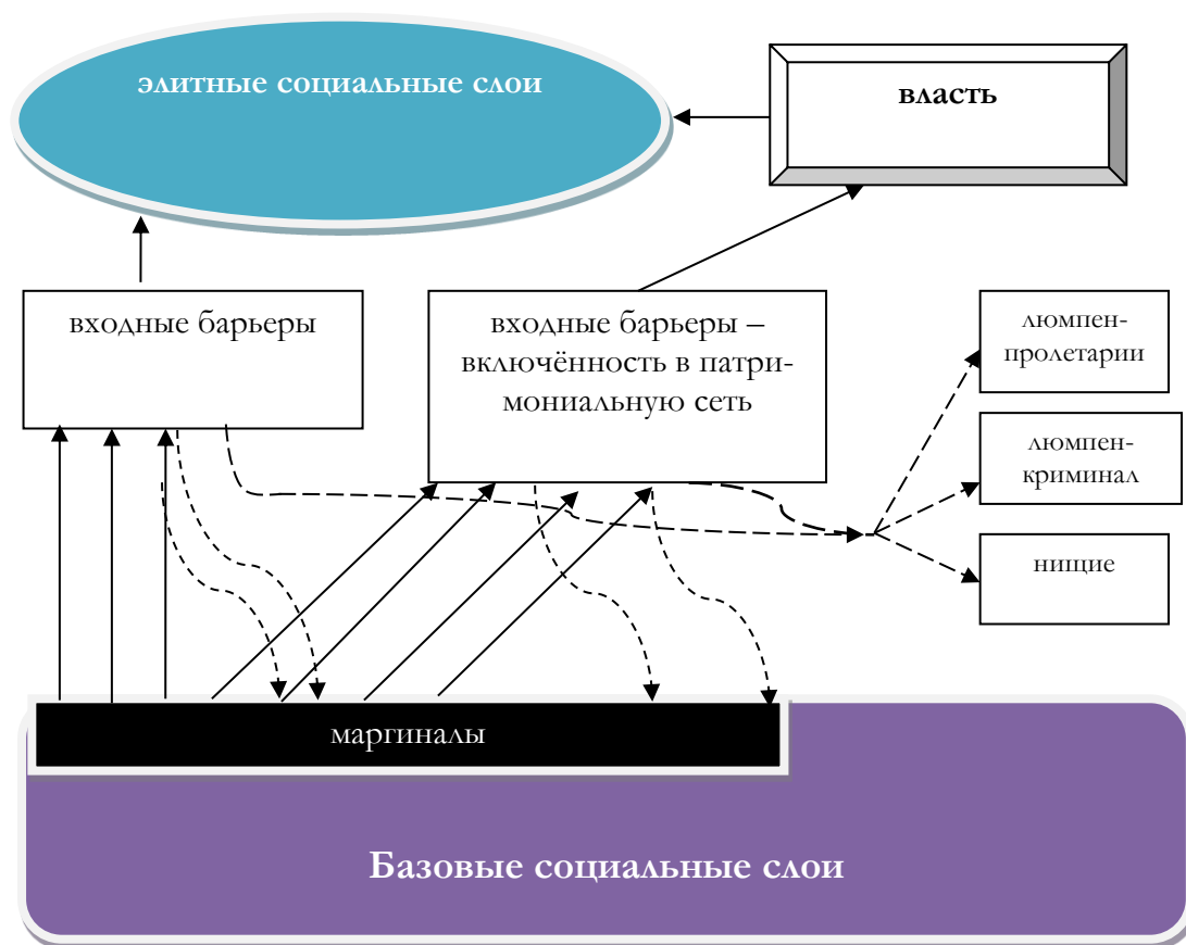
Рис. 5. Модель социальной динамики современной России
