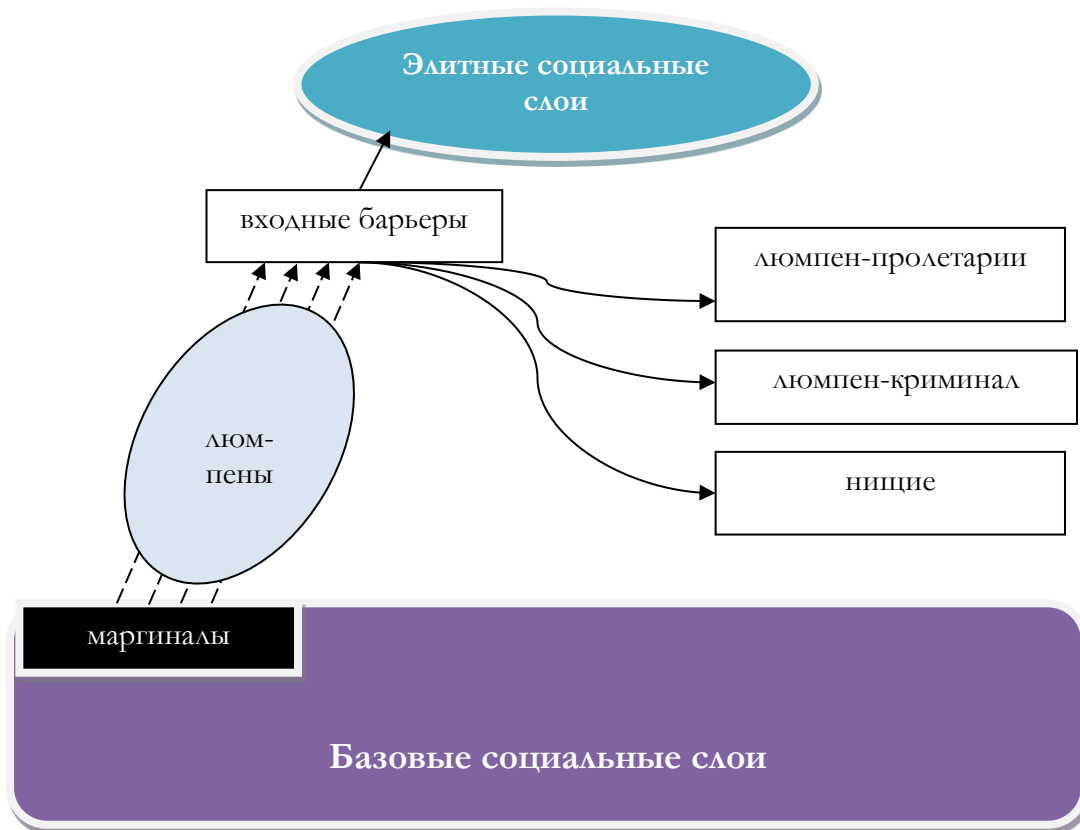
Рис. 1. Базовая модель социальной динамики
