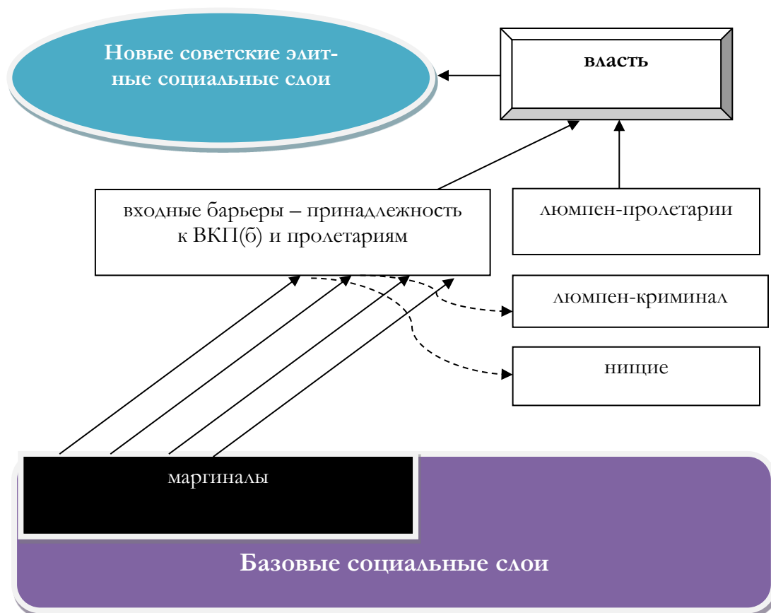
Рис. 3. Модель социальной динамики в Советской России на этапе диктатуры люмпен-пролетариата
