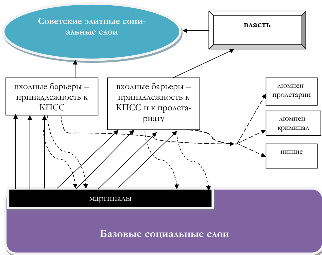
Рис. 4. Модель социальной динамики в Советской России на этапе диктатуры люмпен-номенклатуры
