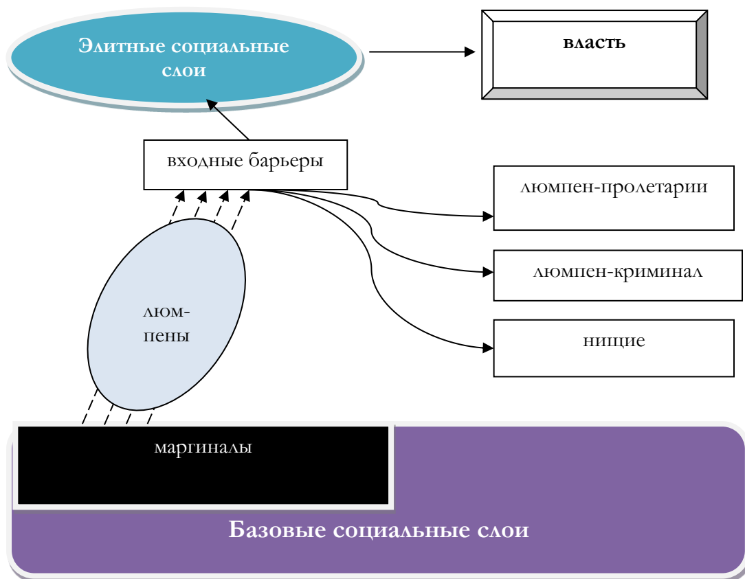
Рис. 2. Модель социальной динамики в царской России до февраля 1917 года
