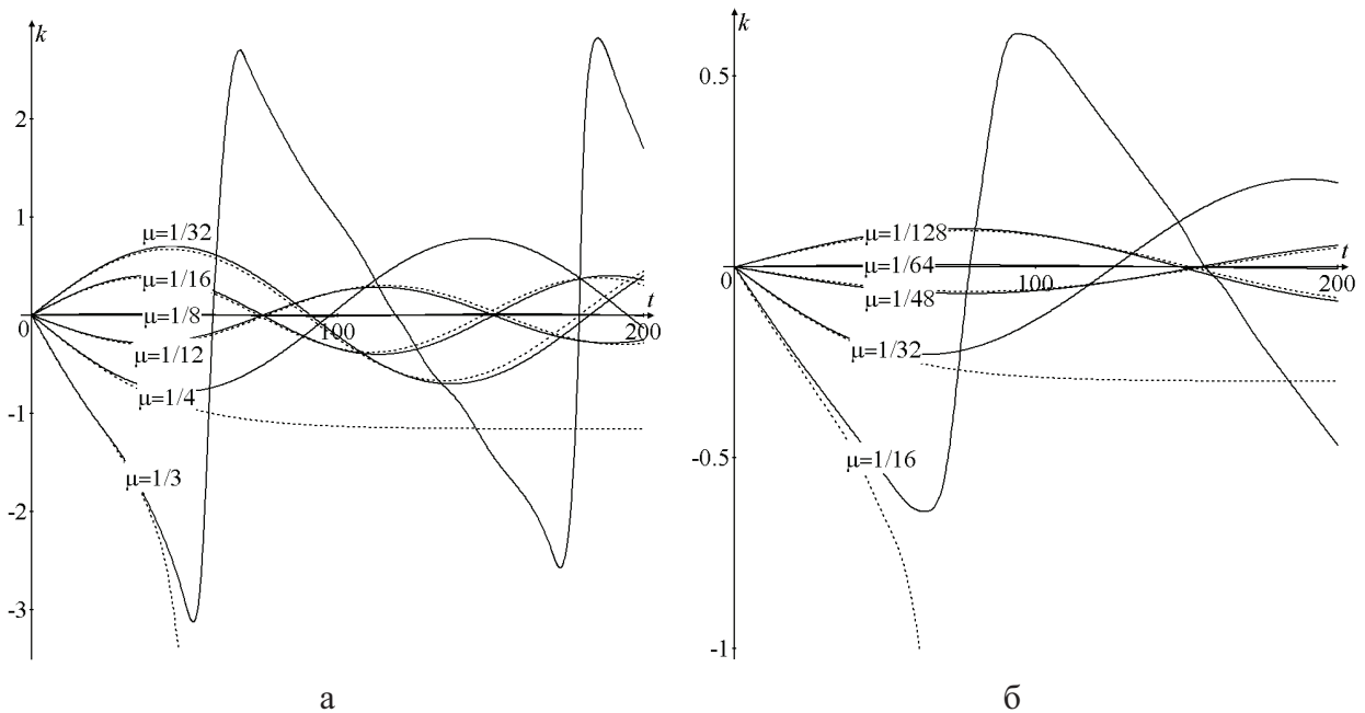
Рис. 8. Волновое число солитона в точке максимума модуля огибающей солитона в зависимости от t при различных значениях величины \mu :
