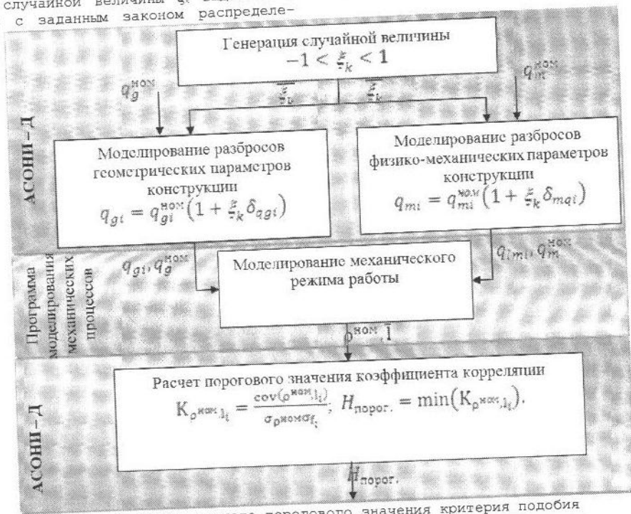
Рис. 1. Метод расчета порогового значения критерия подобия
