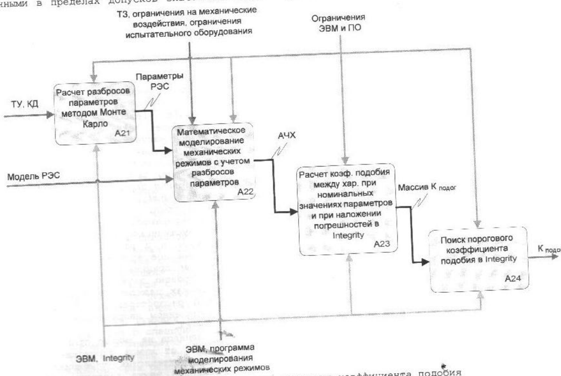
Рис. 2. Расчет порогового значения коэффициента подобия в подсистеме диагностирования БРТУ «Integrity»
